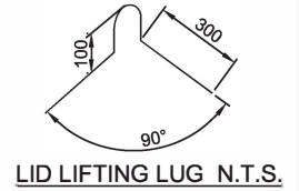
LID LIFTING LUG N.T.S.
