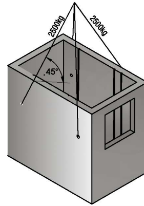
ISOMETRIC VIEW N.T.S.
