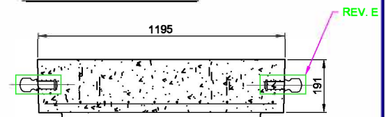
VAULT LID B-B 1:25
