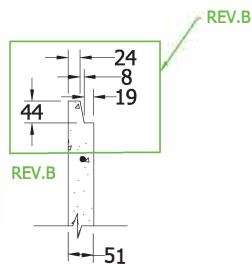
TONGUE & GROOVE DETAIL SCALE 1 : 15
