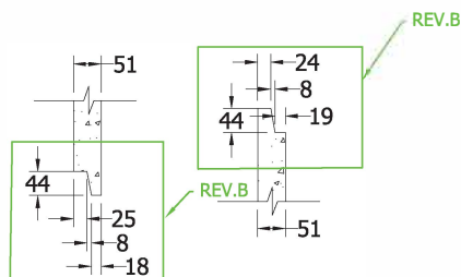
TONGUE & GROOVE DETAIL SCALE 1 : 15
