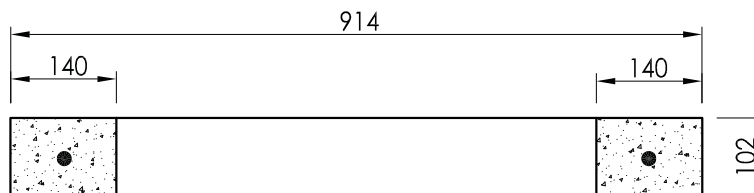
SECTION A-A SCALE : 1:10
