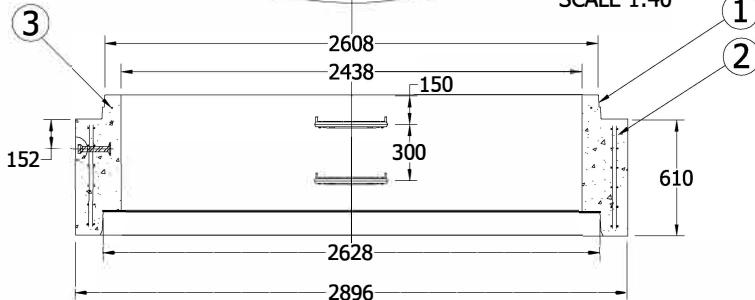
SECTION A-A SCALE 1:40
