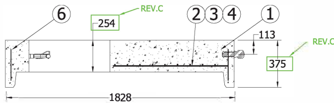
SECTION A-A SCALE 1:20
