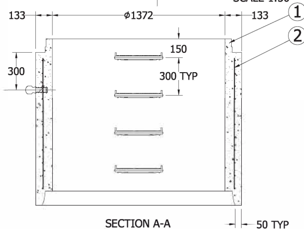
SECTION A-A SCALE 1:30
