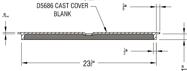
SECTION A - A D5686 COVER N.T.S.
