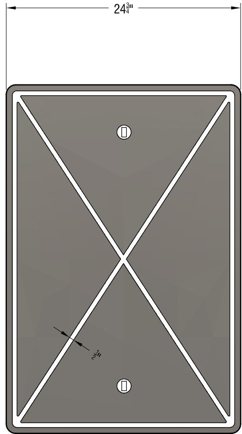
BOTTOM VIEW D5686 COVER N.T.S.
