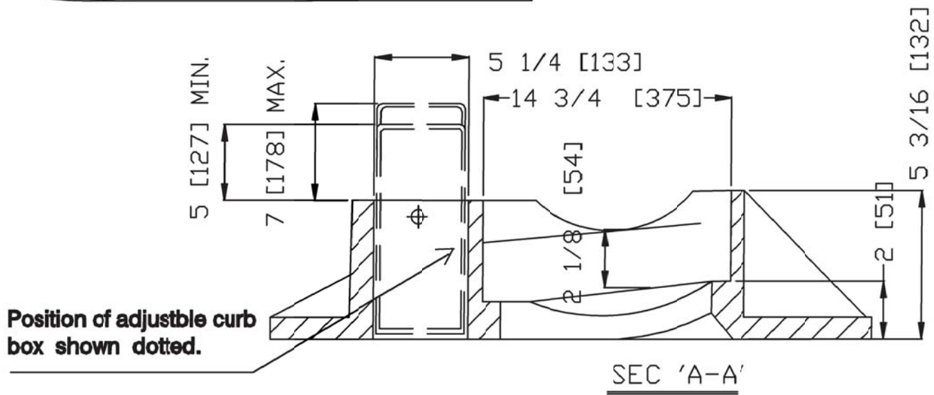
D24A:-Adjustable Frame used with D23-Grates
