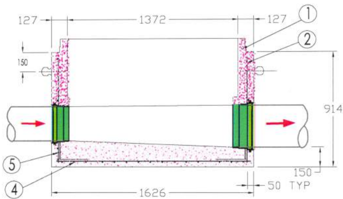
SECTION A-A SCALE 1:30
