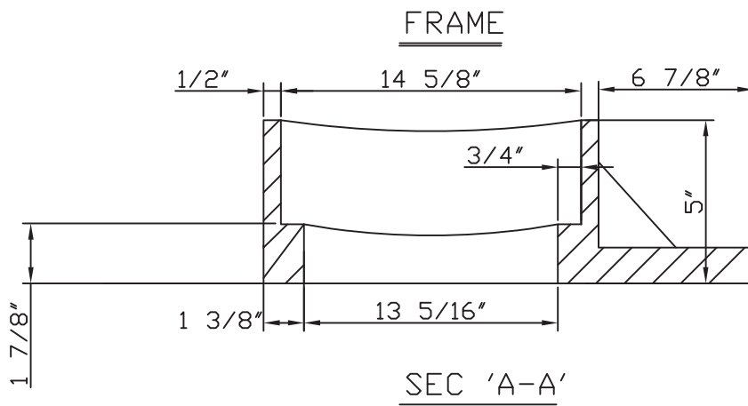
D24D:-D-Frame for D23 Grate
